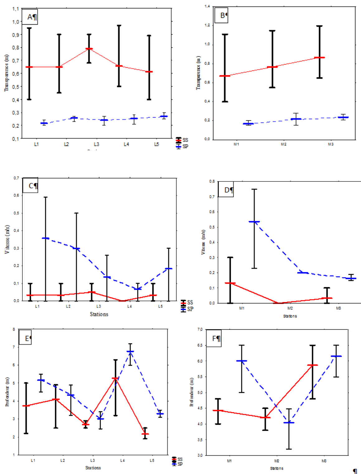
Figure 3 : Variations spatio-saisonnières de la transparence (A et B), de la vitesse de l'eau (C et D) et de la profondeur (E et F) dans les eaux du bassin du Haut-Bandama, d'octobre 2017 à septembre 2018. L1 à L5 = stations de la rivière Lokpoho ; M1 à M3 = Stations du fleuve Bandama
