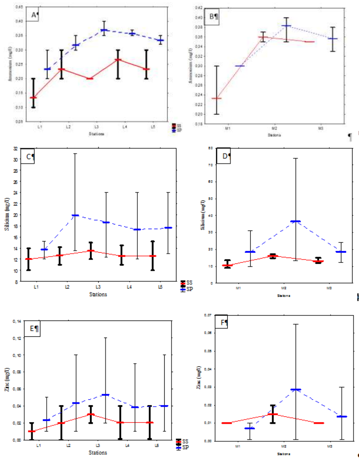
Figure 5 : Variations spatio-saisonnières de l'ammonium (A et B), du potassium (C et D) et du phosphate (E et F) dans les eaux du bassin du Haut-Bandama, d'octobre 2017 à septembre 2018. L1 à L5 = stations de la rivière Lokpo ; M1 à M3 = Stations du fleuve Bandama
