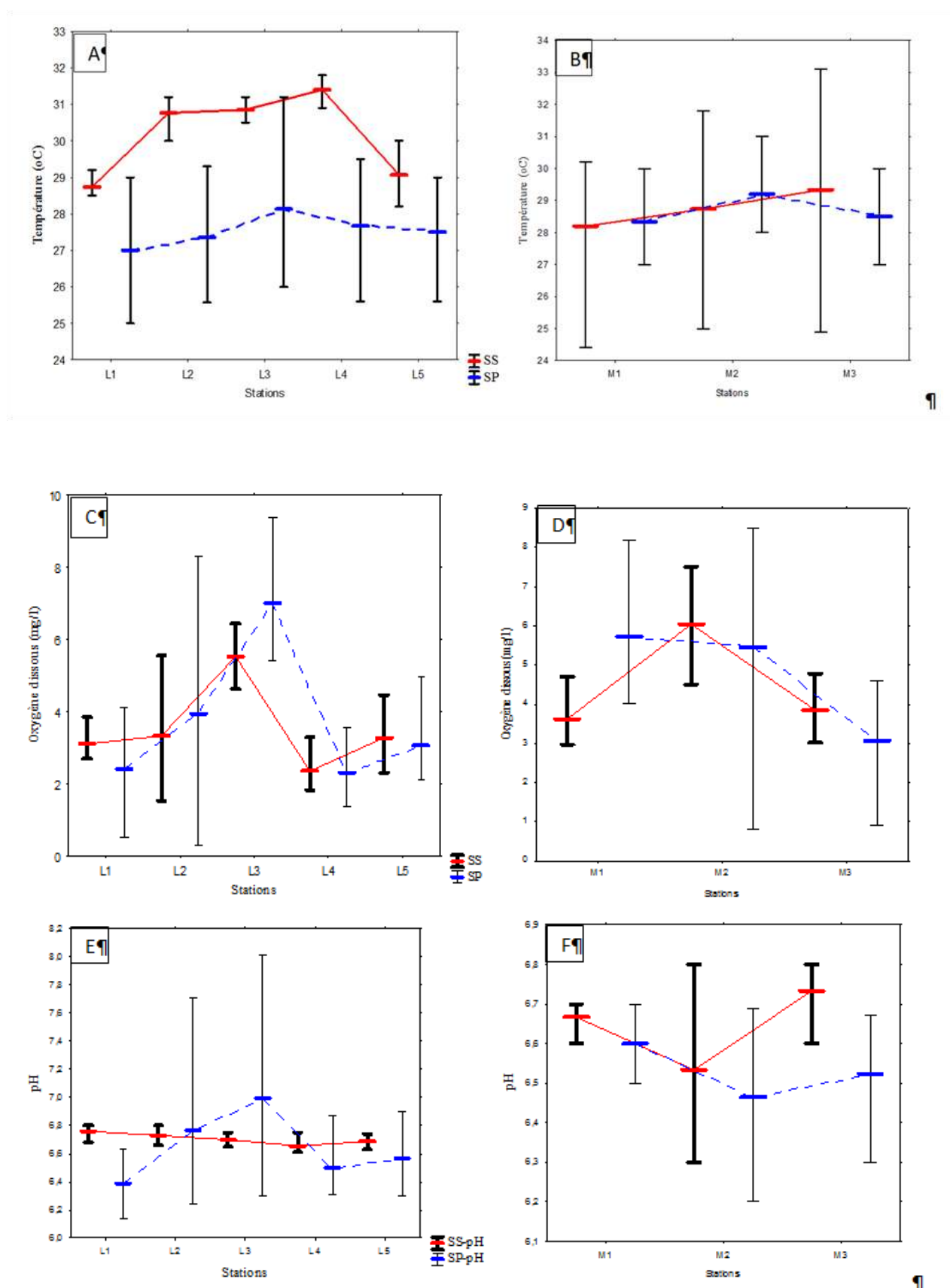
Figure 2 : Variations spatio-saisonnières de la température (A et B), de l'oxygène dissous (C et D) et du pH (E et F) dans les eaux du bassin du Haut-Bandama, d'octobre 2017 à septembre 2018. L1 à L5 = stations de la rivière Lokpoho ; M1 à M3 = Stations du fleuve Bandama.
